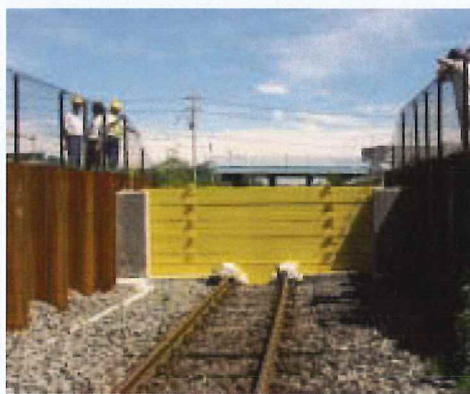
左岸側止水壁
