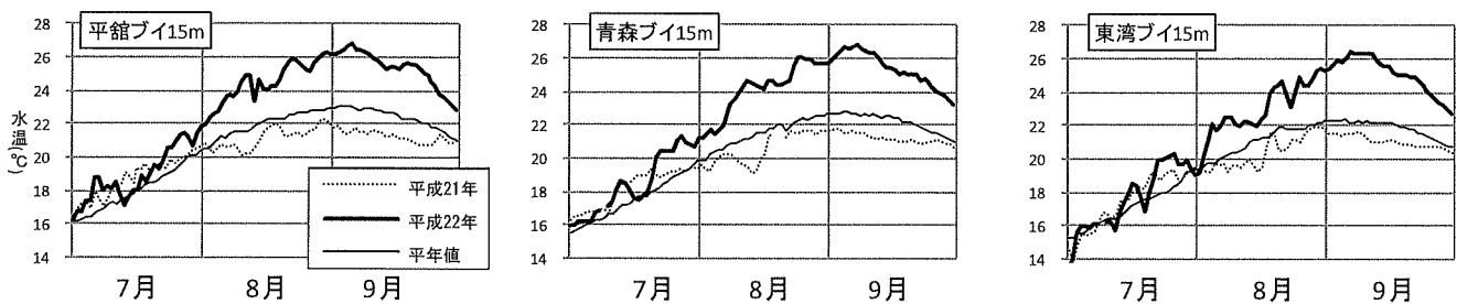
図 1 平成 22 年 7 月～9 月の、水深 15m 層の日平均水温の推移
