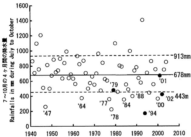
図2 1941年から2004年までの7～10月の4ヶ月間降水量の変化(広島地方気象台における降水量) Fig. 2 Annual changes in total amount of rainfalls during July to October at Hiroshima Local Meteorological Observatory.
