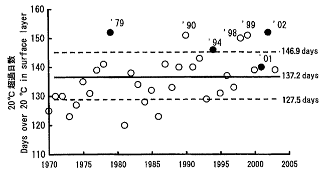
図1 1970年から2004年までの水温20℃超過日数の経年変化(水産海洋技術センター地先の表層水温)
