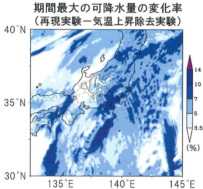
図3 可降水量（鉛直方向に積算した水蒸気量）の変化率 再現実験の期間最大の可降水量から気温上昇除去実験（1980年以降）の期間最大の可降水量を引いた図。気温上昇除去実験からの増加率（%）として描画。
