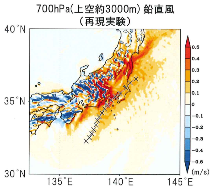
図4 再現実験の鉛直風 台風第19号が関東に接近した際の上空約3000m（700hPa）の鉛直風。令和元年10月12日15時から13日午前6時までの平均値。赤色は上昇流、青色は下降流を示す。×印は一つの再現実験で計算された台風の中心位置。
