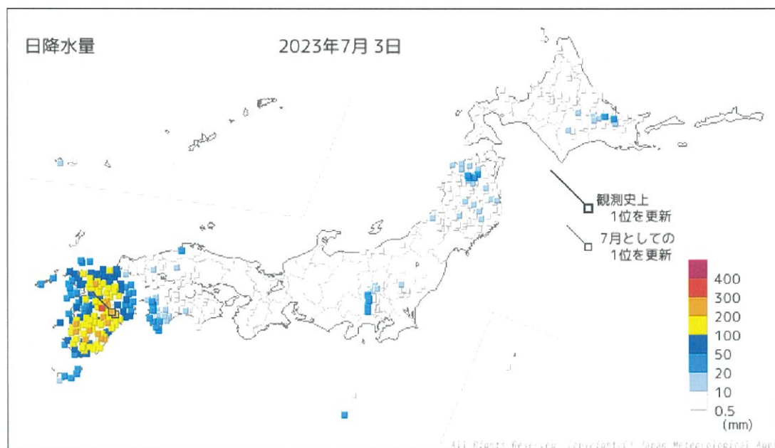
日降水量分布図（7 月 3 日）
