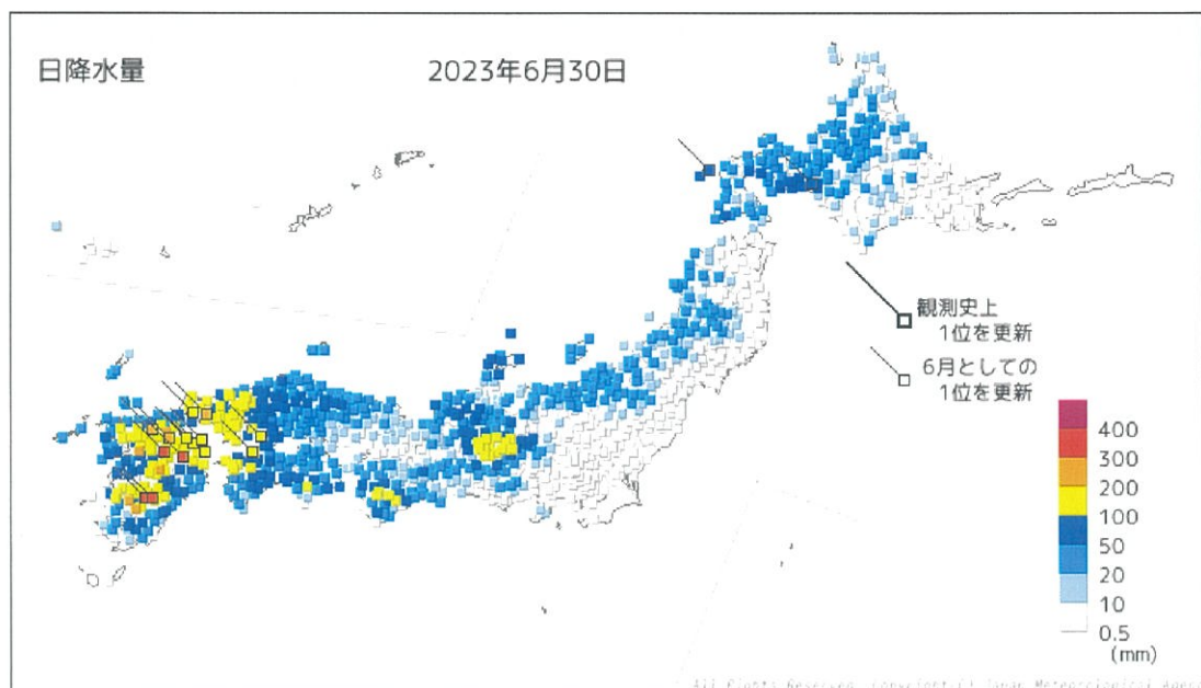
日降水量分布図（6 月 30 日）
