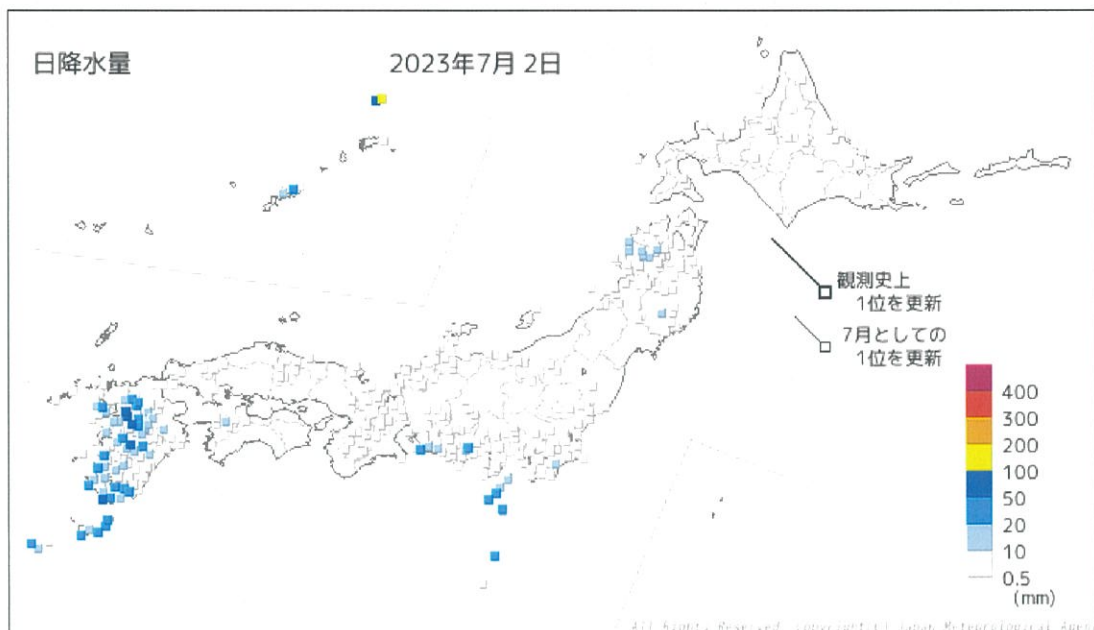
日降水量分布図（7月2日）
