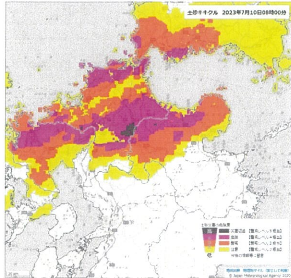
土砂キキクル
