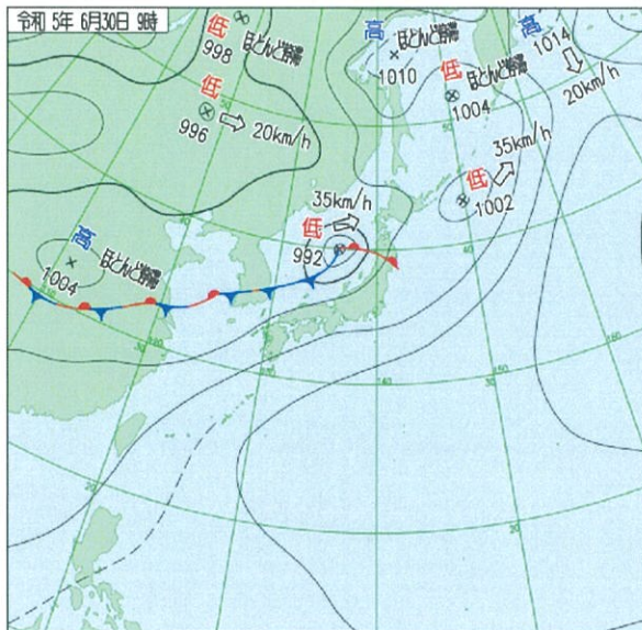
地上天気図（6 月 30 日 09 時）
