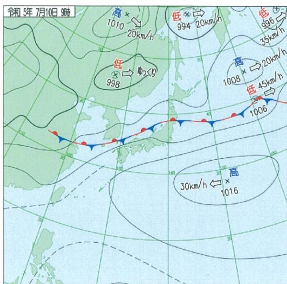
地上天気図 (7 月 10 日 09 時)
