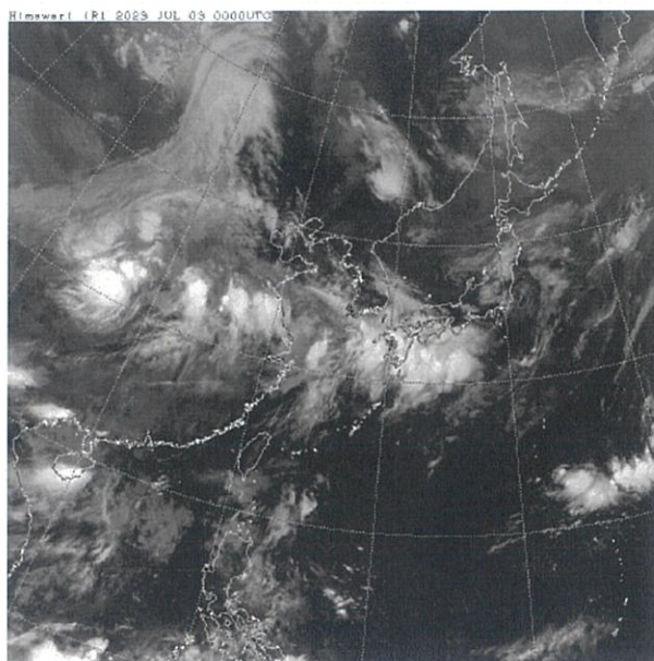
衛星赤外画像（7 月 3 日 09 時）
