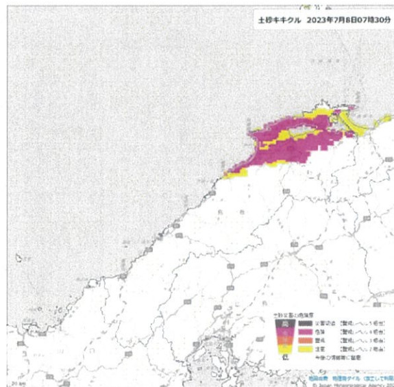
土砂キキクル
