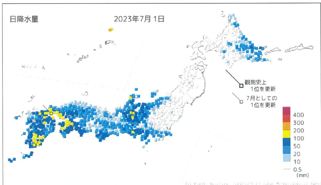
日降水量分布図（7月1日）
