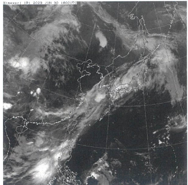
衛星赤外画像（7月1日03時）
