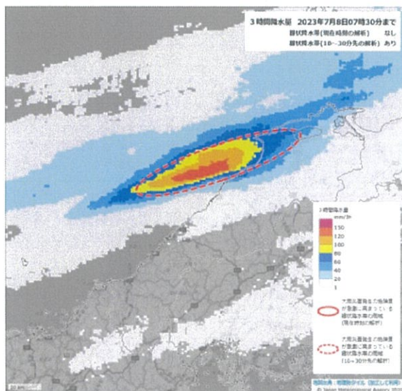
3時間降水量（解析雨量） mm
