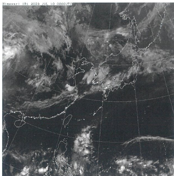
衛星赤外面像 (7 月 10 日 09 時)
