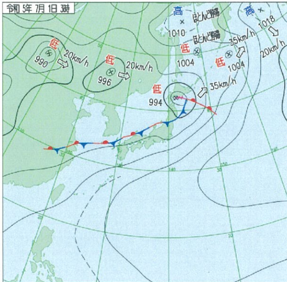
地上天気図（7月1日03時）
