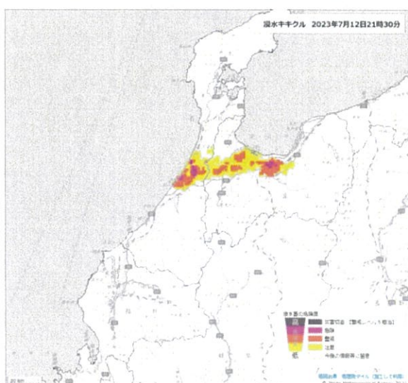
浸水キキクル
