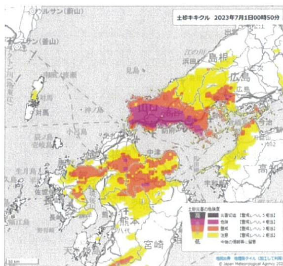
土砂キキクル
