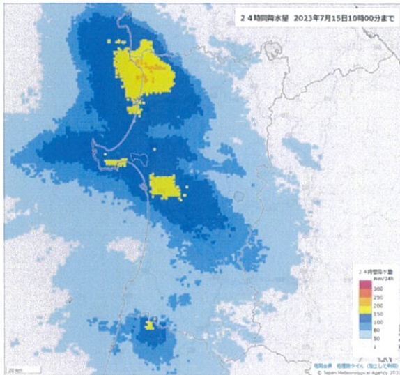
24 時間降水量（解析雨量） mm
