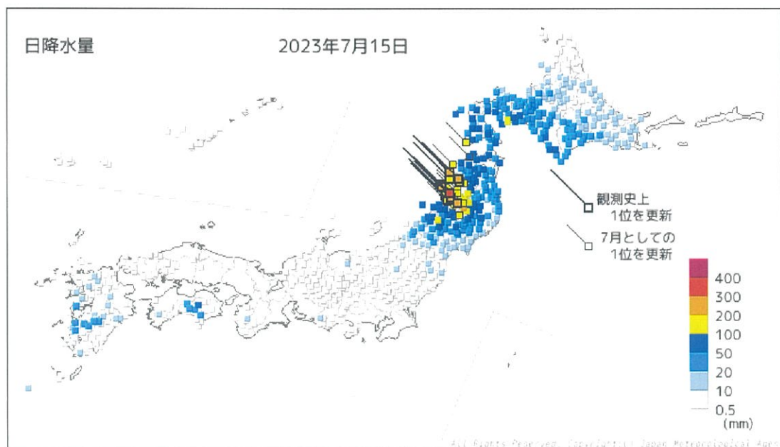
日降水量分布図 (7 月 15 日)
