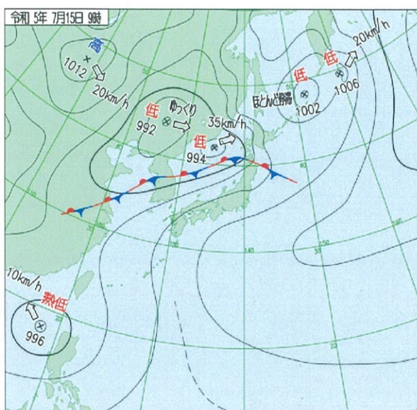
地上天気図 (7 月 15 日 09 時)
