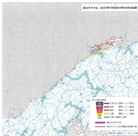
洪水キキクル
