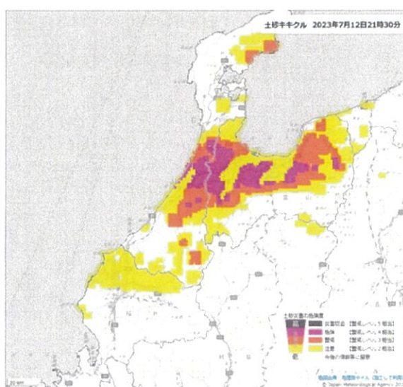
土砂キキクル
