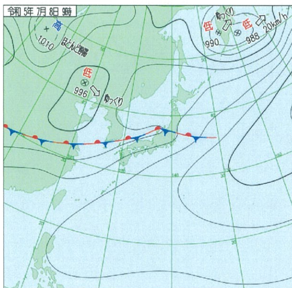
地上天気図（7月8日09時）
