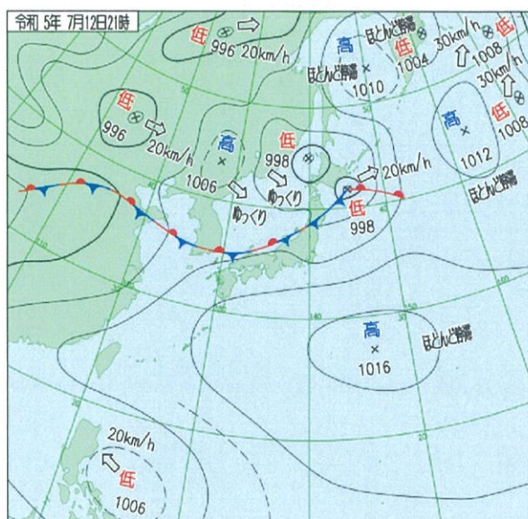
地上天気図（7月12日21時）
