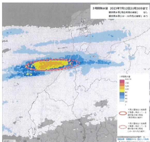
3 時間降水量（解析雨量） mm
