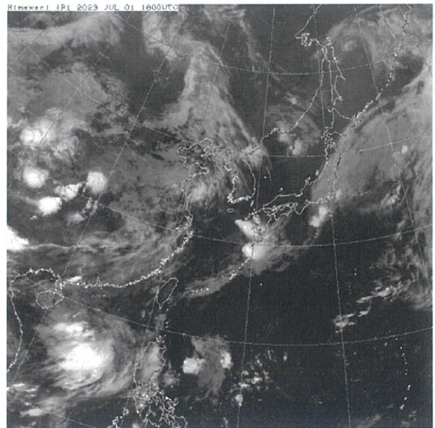
衛星赤外画像（7月2日03時）
