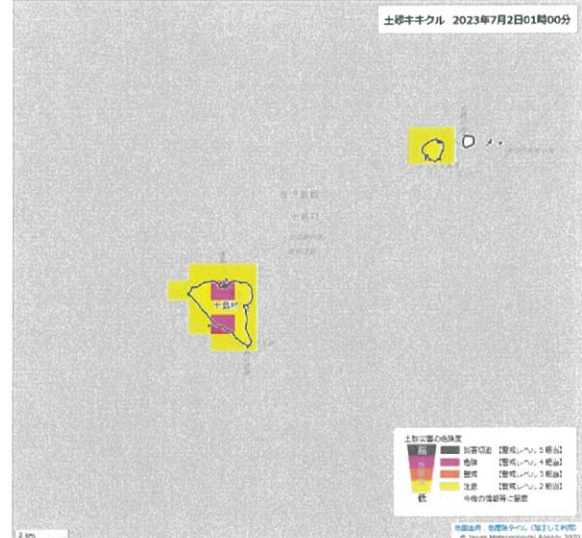
土砂キキクル（宝島付近を拡大）
