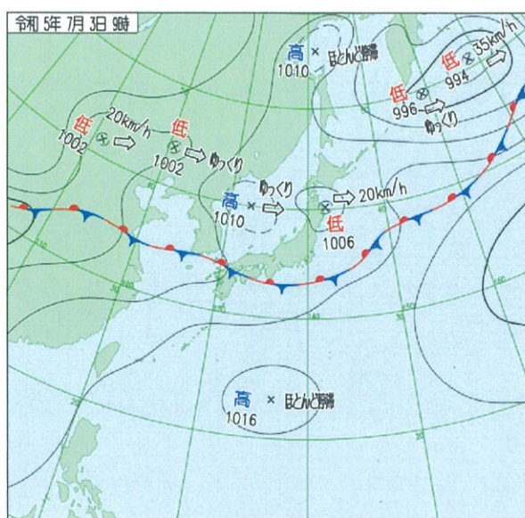
地上天気図（7 月 3 日 09 時）
