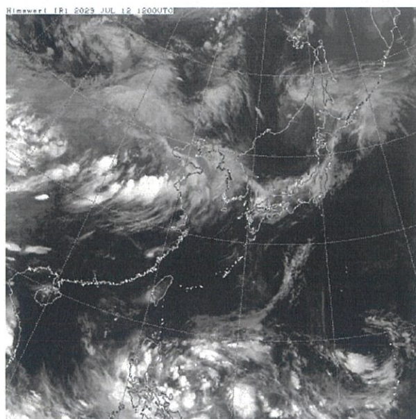
衛星赤外画像（7月12日21時）
