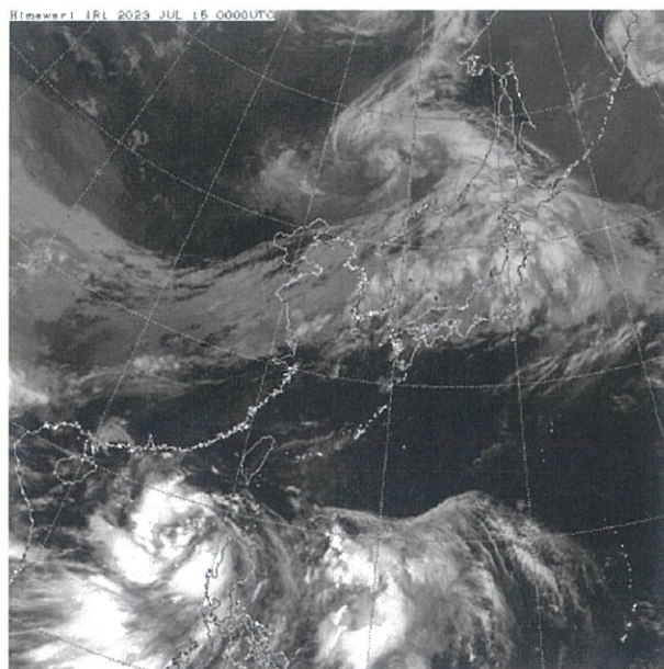
衛星赤外面像 (7 月 15 日 09 時)
