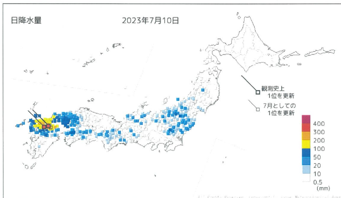
日降水量分布図 (7 月 10 日)
