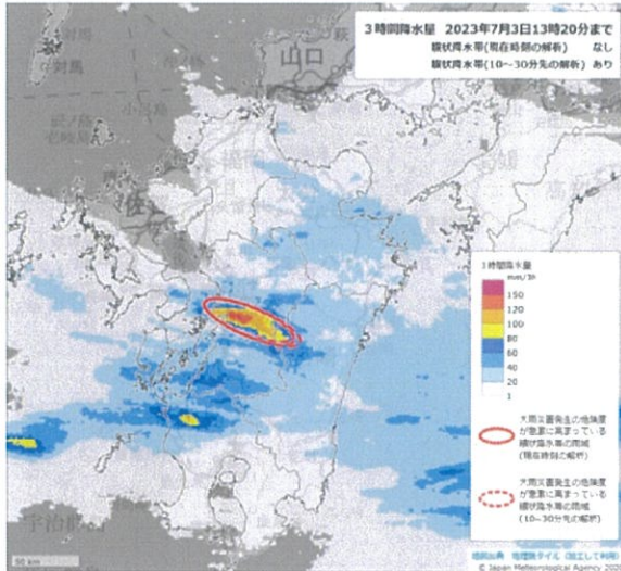
3時間降水量（解析雨量） mm
