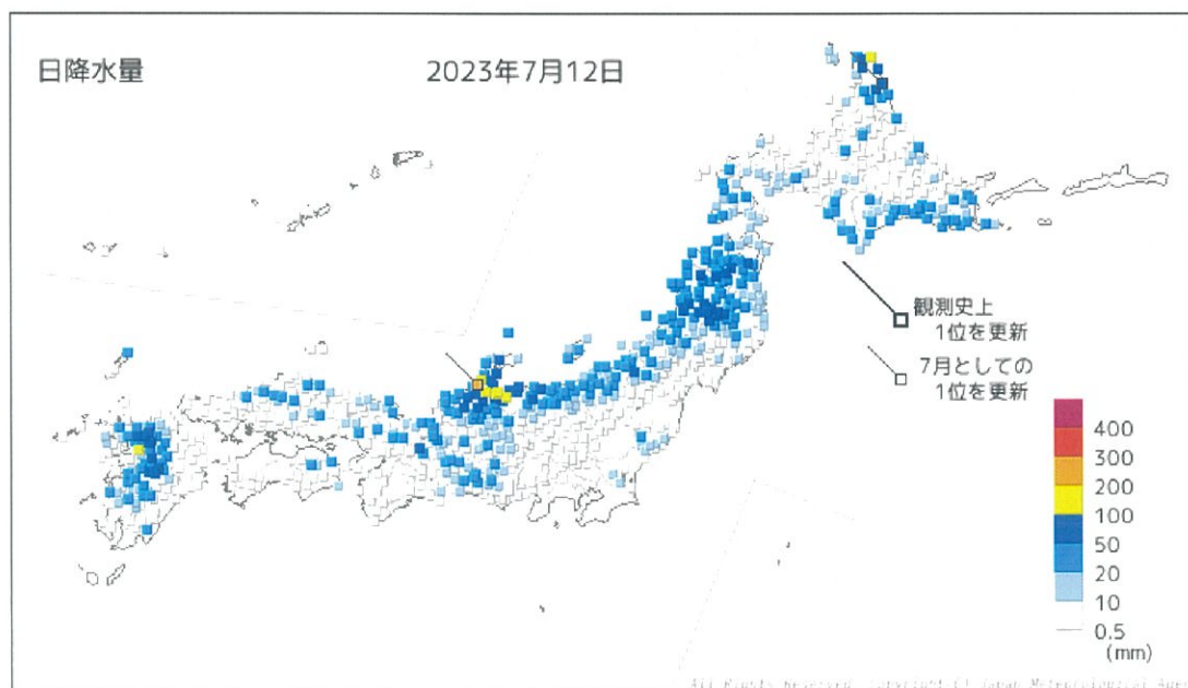
日降水量分布図（7月12日）
