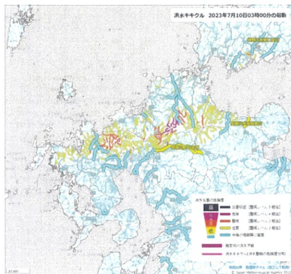
洪水キキクル
