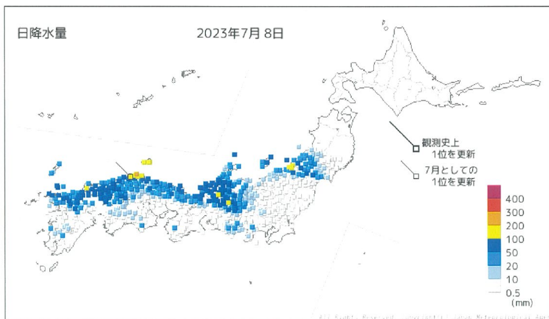
日降水量分布図（7月8日）
