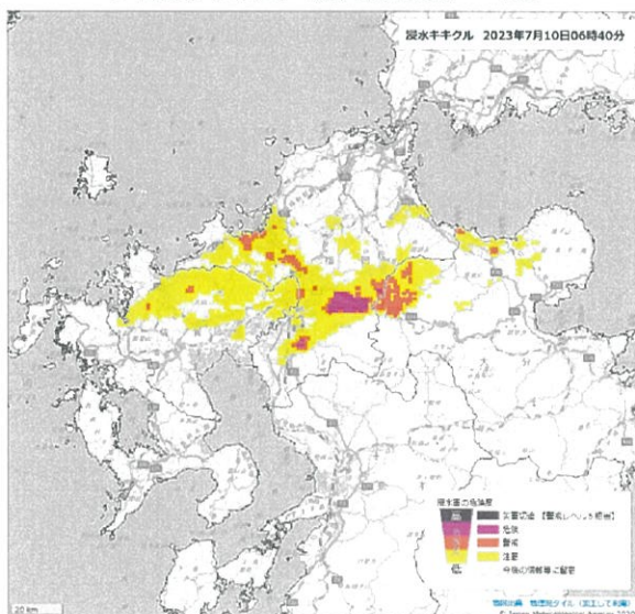
浸水キキクル
